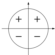
\sin の正負
