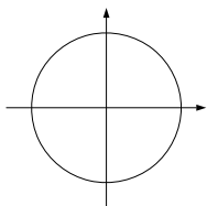
\cos の正負
