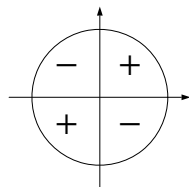
\tan の正負
